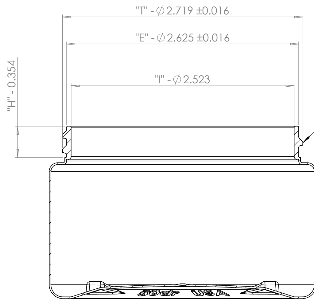
SECTION A-A
